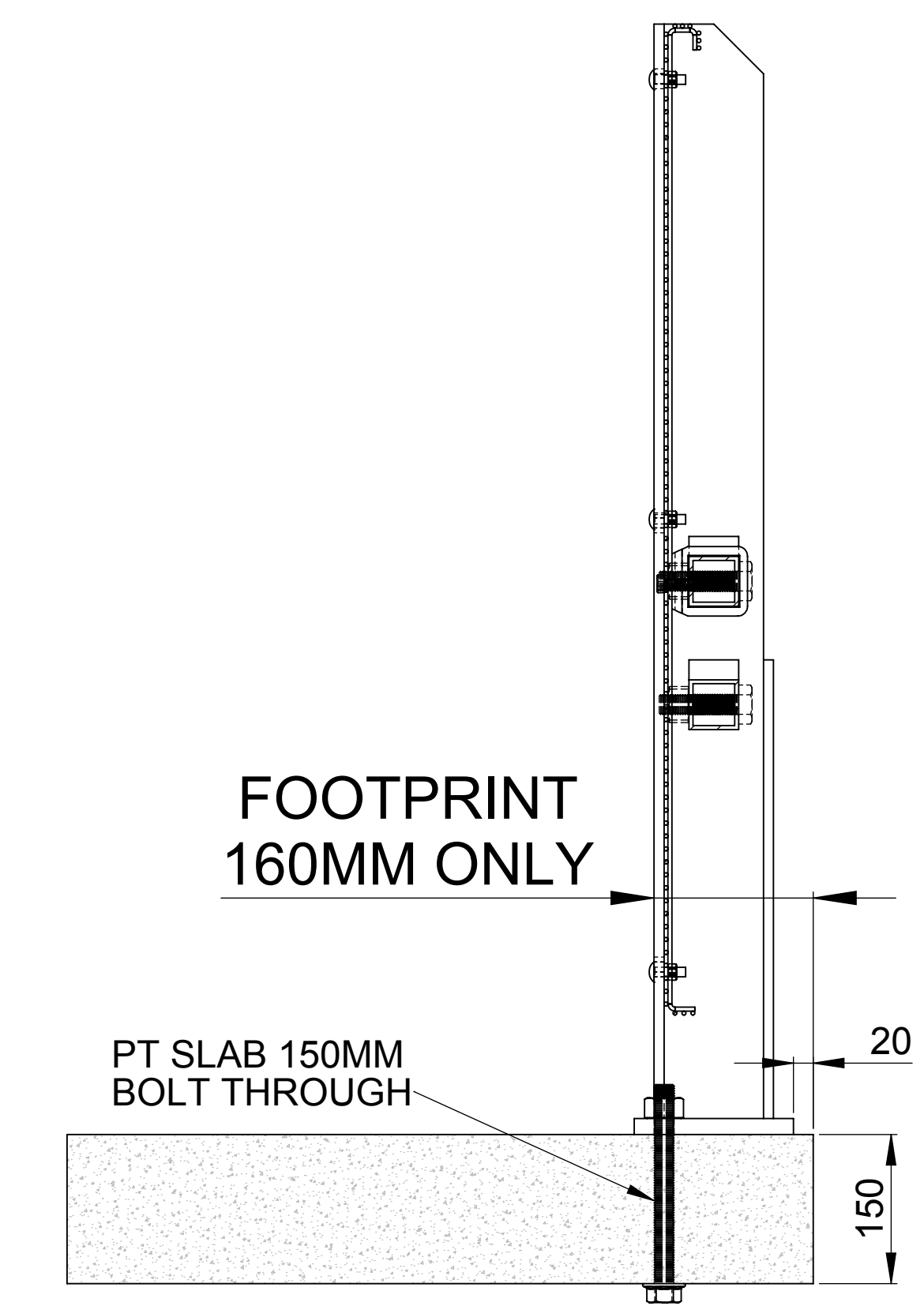
SECTION A-A
