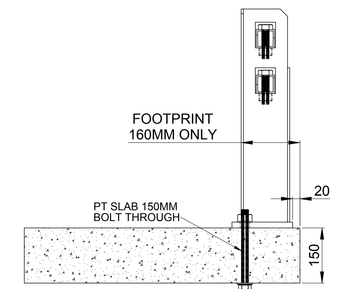
SECTION A-A
